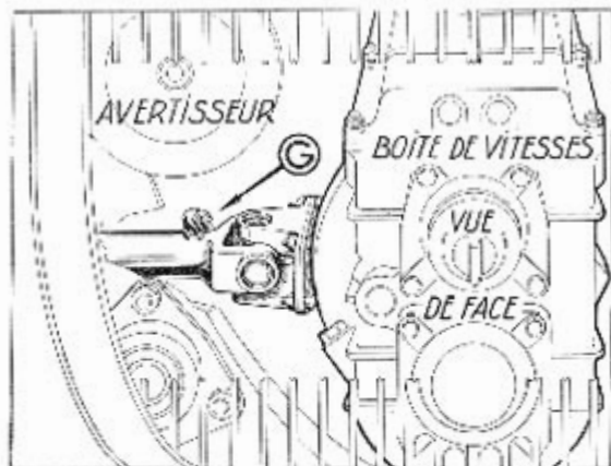
Fig. 13. — GRAISSEUR DES CANNELURES DE CARDAN SUR 11 B (1).
