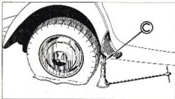
Fig. 6. — POSITION DU CRIC A L'ARRIERE.
