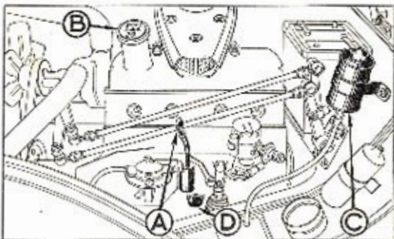
Fig. 1. — JAUGE D'HUILE (A). — ORIFICE DE REMPLISSAGE (B). — RÉSERVOIR DU LIQUIDE POUR FREINS (C).
