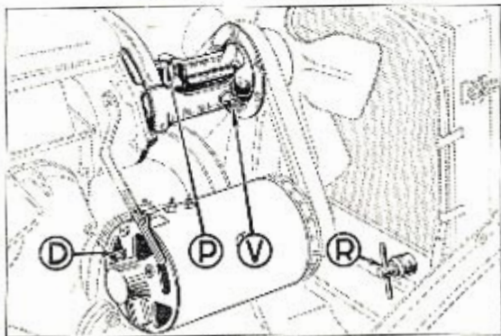
Fig. 16. — DYNAMO PARIS-RHONE.
