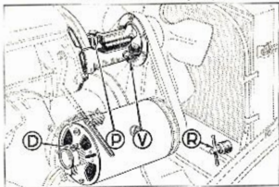
Fig. 15. — DYNAMO DUCELLIER.
