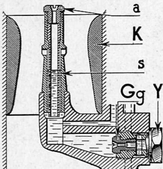
Fig. 31 — Montage 21 en coupe.
