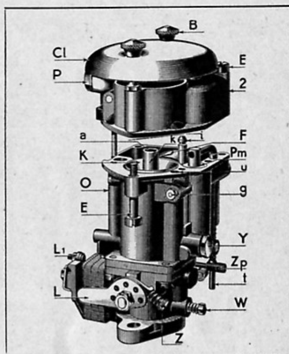
Fig. 20. — Vue extérieure, démonté
