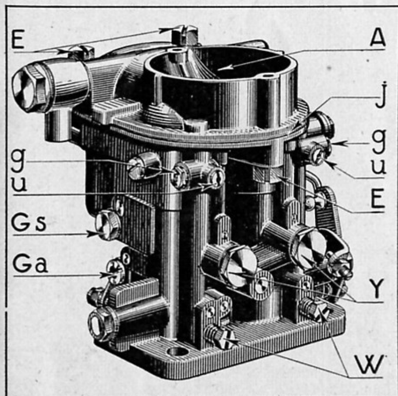
Fig. 24 — Solex double-corps inversé type 30 FFIAP à bistarter. Pompe mécanique. Montage 21. Démonté.
