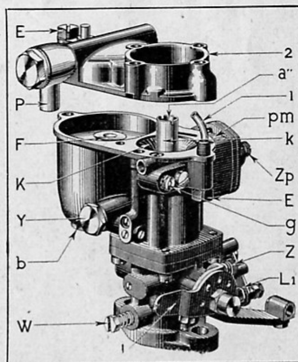
Fig. 15. — Vue extérieure démonté
