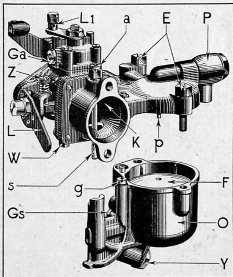
Fig. 4. — Solex horizontal type AHD à bistarter. Montage 22. Ralenti à réglage d'essence.
