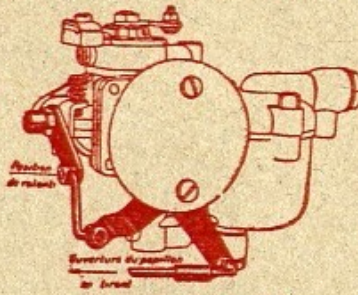
HD cuve à droite En tirant
