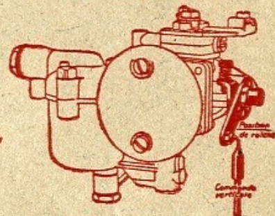
HBFG cuve à gauche Commande verticale
