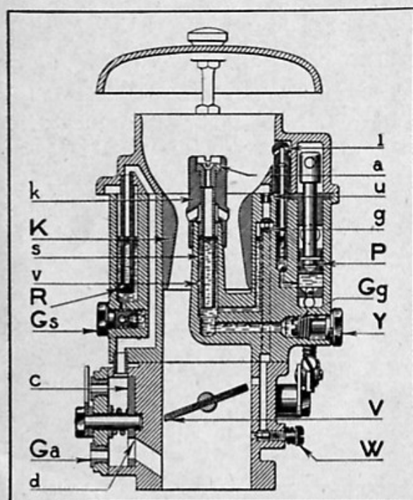
Fig. 19. — Coupe du SOLEX inversé type 35 FILP (à starter - Montage 20 - Ralenti à réglage d'essence - Pompe mécanique)
