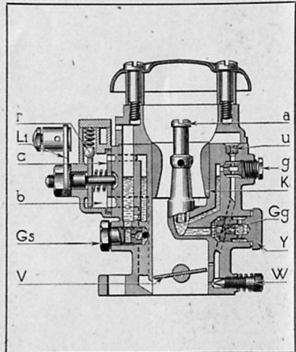
Fig. 11. — [Coupe longitudinale
