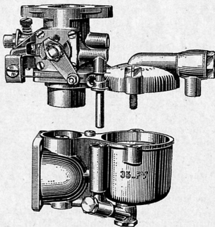
Fig. 7. — Carburateur FV à starter, démonté.
